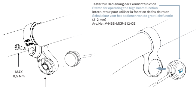
MSH22 Halter • Mount • Support • Bevestigingsbeugel Kompatibel mit Supernova Taster für die Fernlichtfunktion. Compatible with Supernova switch for high beam function. Compatible avec l'interrupteur Supernova pour la fonction de feu de route. Compatibel met Supernova-schakelaar voor grootlichtfunctie. Art. No.: W-MSH22
